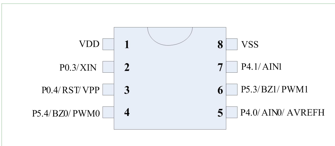
图 1 HS26P11- SOP8
