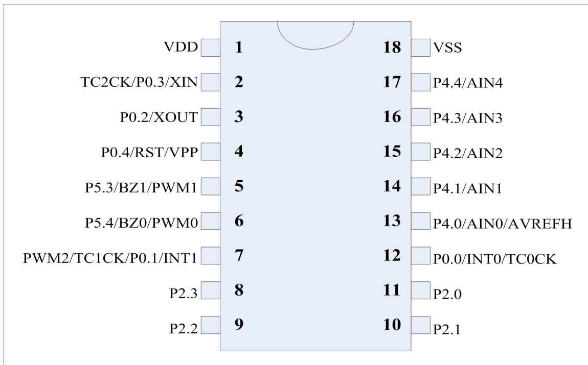
图 4 管脚分配 SOP18/DIP18
